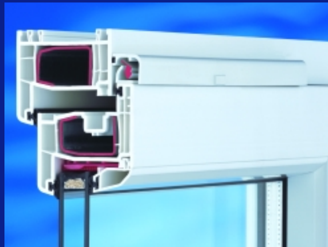
Klappe geöffnet
